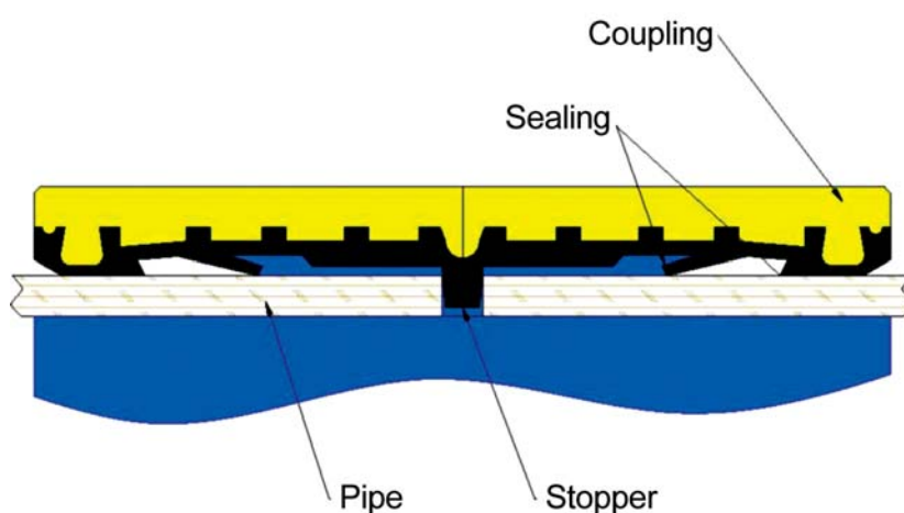
איור מס' 12 | חתך מחבר פעמון מסוג עפרה
